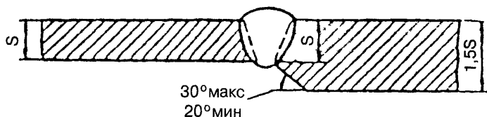
Рис. 1. Конструктивные размеры разделки кромок и сварных швов разнотолщинных труб (до 1,5 толщины стенки)
