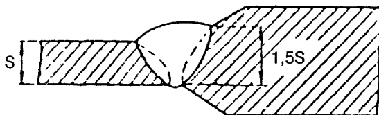
Рис. 2. Подготовка кромок патрубков арматуры при непосредственном соединении их с трубами
