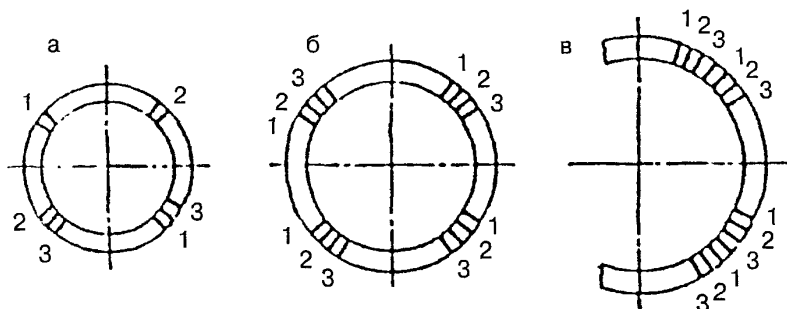
Рис. 3. Схема вырезки образцов для механических испытаний
