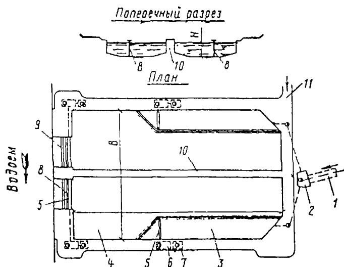
Рис. 5. Схема пруда-отстойника на сопряжении с водоёмом
