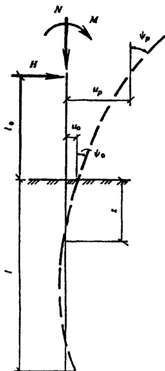
Схема нагрузок на сваю
