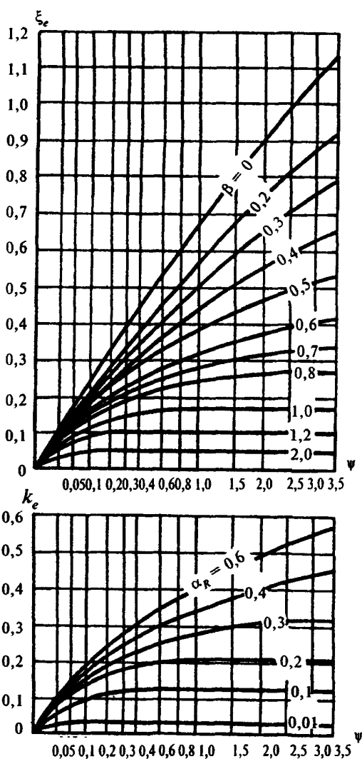
Черт. 2. Графики для определения коэффициентов \xi_e и k_e
