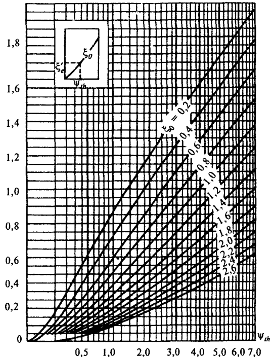
Черт. 6. Графики для определения коэффициента \xi'_e
