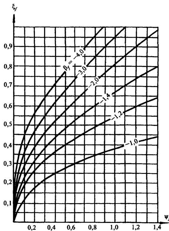
Черт. 1. Графики для определения коэффициента \beta_f
