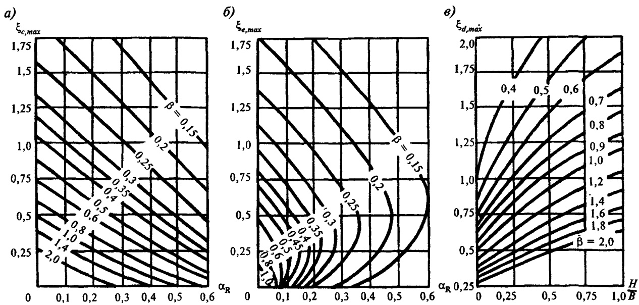
Черт. 3. Графики для определения коэффициентов:
