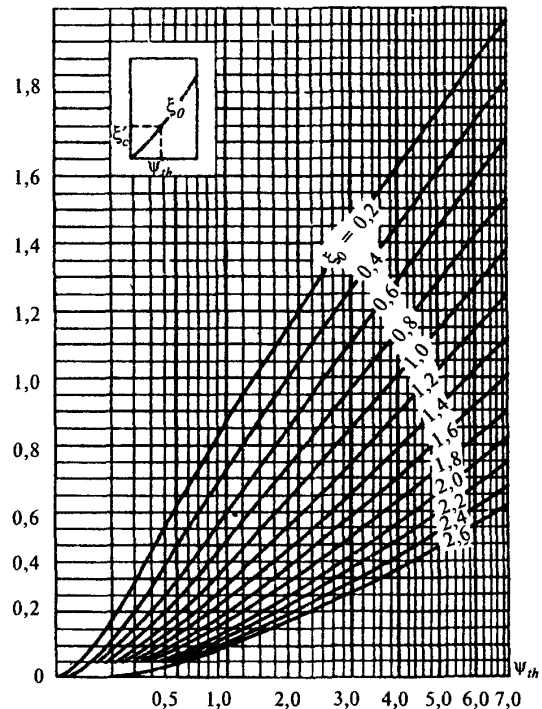
Черт. 5. Графики для определения коэффициента \xi'_c
