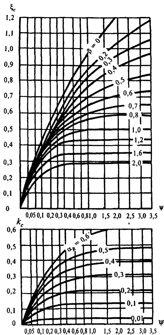
Черт. 1. Графики для определения коэффициентов \xi_c и k_c
