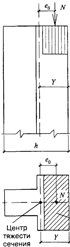
Рис. 5. Внецентренное сжатие
