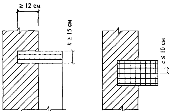
Рис. 13. Железобетонные распределительные плиты
