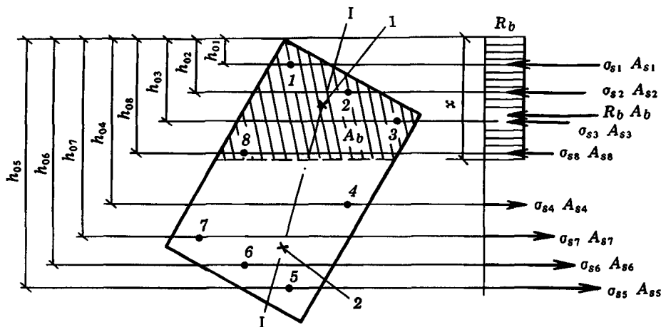
Черт. 1. Схема усилий и эпюра напряжений в сечении, нормальном к продольной оси железобетонного элемента, при расчете его по прочности
