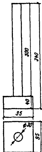
РИС. 8. СТАЛЬНАЯ БОЛВАНКА ДЛЯ ТРАМБОВАНИЯ
