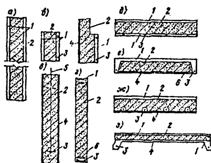
РИС. 1. ЭЛЕМЕНТЫ ИЗ АРБОЛИТА И БЕТОНА
