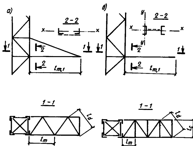
Рис. 21. Схемы траверс
