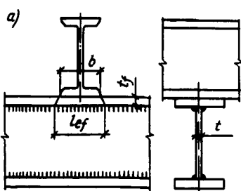
Рис. 5. Схемы для определения длины распределения нагрузки на балку
