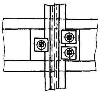
Черт. 6. Прикрепление рельсов к полушпалам
