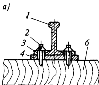
Черт. 4. Прижим для при- крепления рельсов к полушпа- лам шурупами
