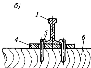
Черт. 5. Прижим облегченный для крепления рельсов к полушпалам шурупами
