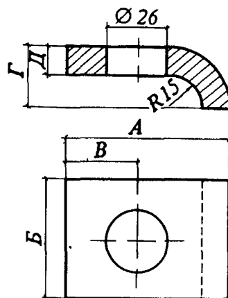
Черт. 5. Прижим облегченный для крепления рельсов к полушпалам шурупами
