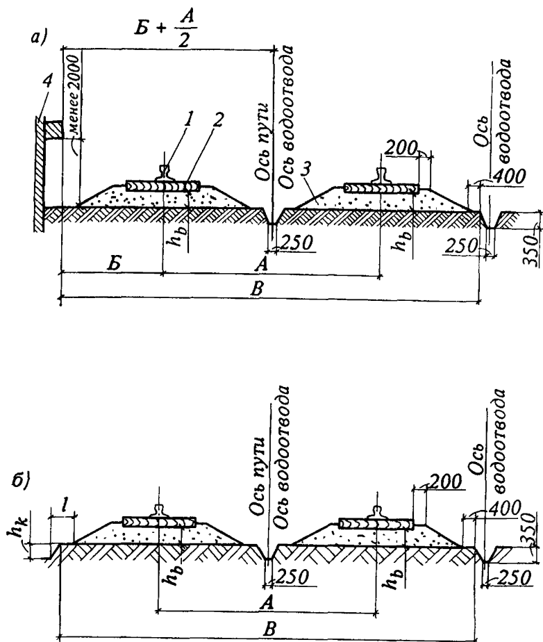
Поперечные профили рельсового пути
