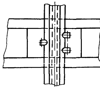
Черт. 6. Прикрепление рельсов к полушпалам
