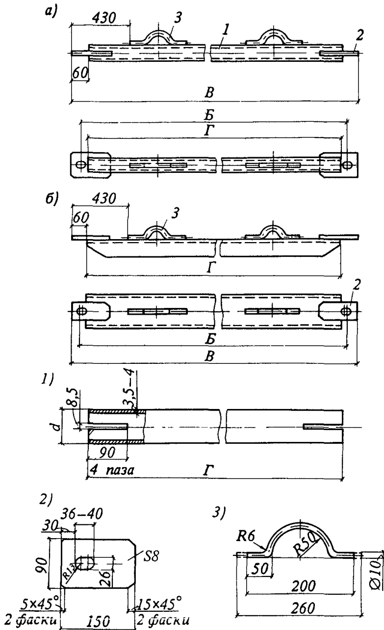
Черт. 11. Стяжки и детали прикрепления стяжек к инвентарным секциям рельсовых путей с железобетонными балками
