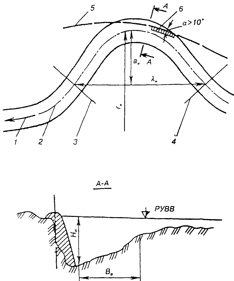
Рисунок Т.1 — К определению радиуса кривизны потока r_w : 1—направление течения; 2—ось русла; 3, 4—конец и начало излучины; 5, 6—трасса и ее входной участок
