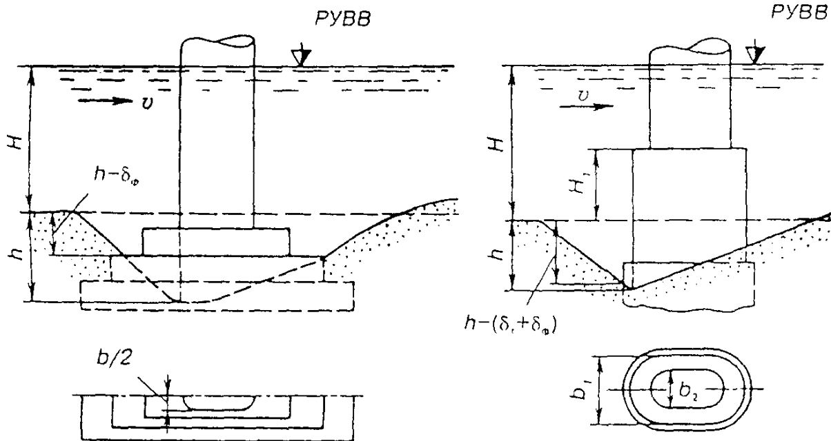
Рисунок 5.2 — Схемы опор на массивном фундаменте: а — с постоянной шириной в пределах глубины потока; б — с переменной шириной в пределах глубины потока
