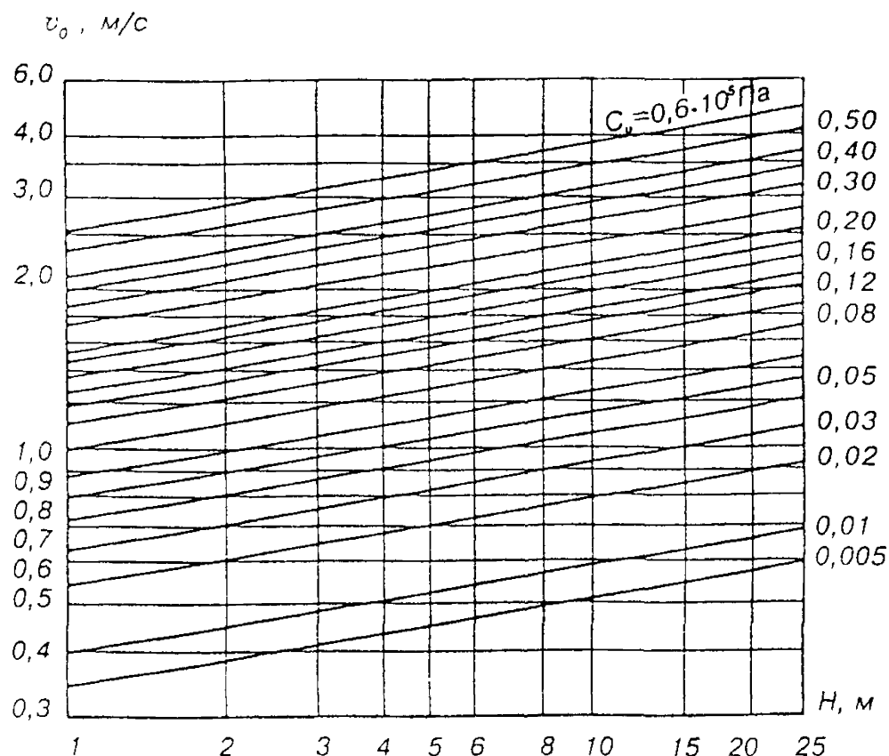
Рисунок А.2 — График для определения размывающей скорости связных грунтов при коэффициенте абразивности \varepsilon=1,0 и коэффициенте шероховатости n=0,03
