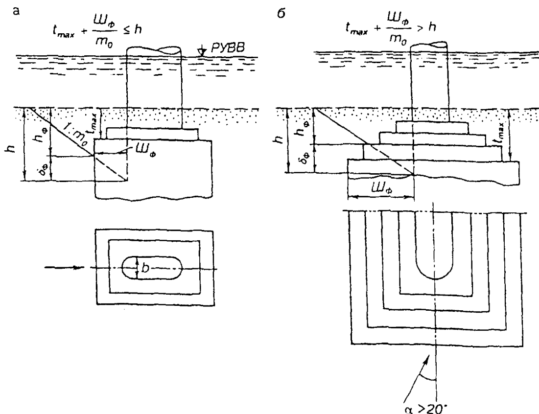
Рисунок Е.1 — К определению глубины уменьшения размыва \delta_{\text{ф}} за счет массивного фундамента в грунтах с одинаковыми физико-механическими свойствами:
