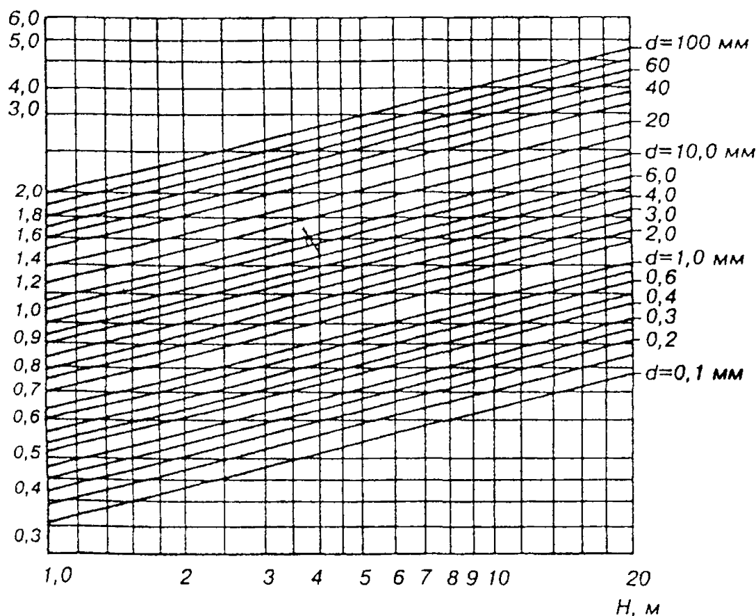
Рисунок А.1 — График для определения размывающей скорости несвязных грунтов
