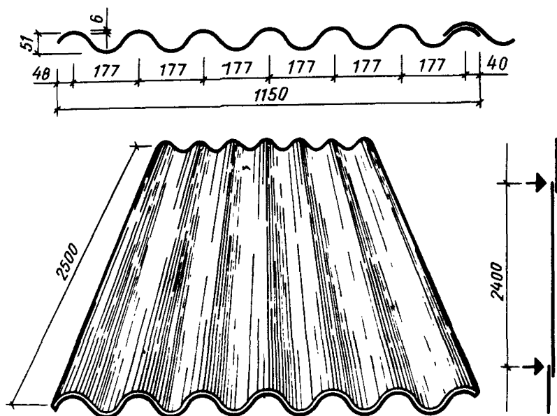
Рис. 3. Асбестоцементные волнистые листы высокого профиля 51/177
