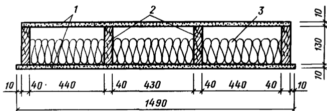
Рис. 2. Поперечное сечение плиты 1 -- асбестоцементные плоские листы; 2 -- доски; 3 -- утеплитель
