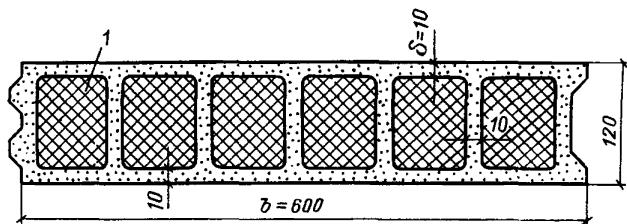
Рис. 8. Поперечное сечение экструзионной панели 1 -- утеплитель
