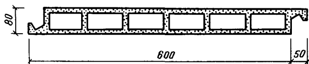
Рис. 13. Поперечное сечение плиты
