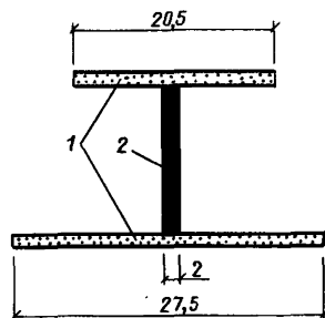
Рис. 7. Расчетное сечение панели 1 -- асбестоцементная обшивка; 2 -- алюминиевый каркас
