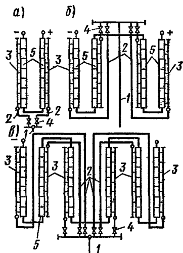
Рис. 5. Схема ввода электролита в коллекторы электролизной установки, обладающая минимальными токами утечки
