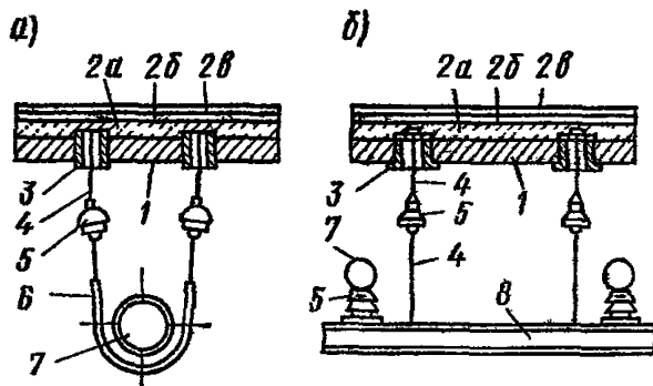
Рис. 3. Пример подвесок типа шпильки для крепления технологических трубопроводов
