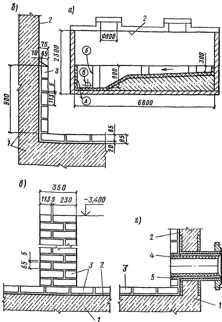
Рис. 2. Усреднитель хромосодержащих стоков
