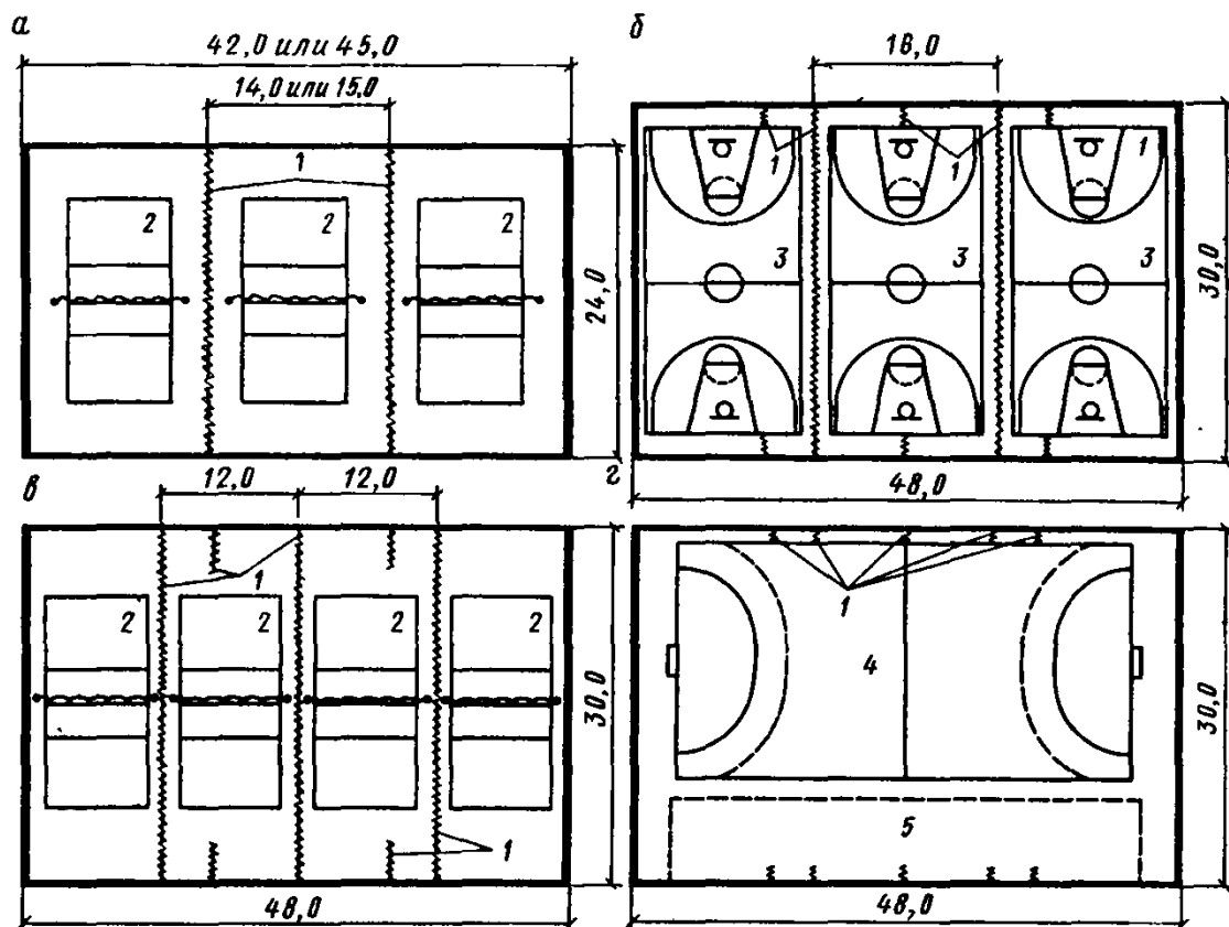
Рис. 2. Варианты схем планов деления залов на секции (размеры в метрах) а — план зала размером 42 \times 24 м (или 45 \times 24 м) с делением его на три секции для учебно-тренировочных занятий по волейболу, б — план зала размером 48 \times 30 м при делении его на три секции для занятий по баскетболу, в — вариант деления зала 48 \times 30 м на четыре секции для занятий по волейболу; г — план зала размером 48 \times 30 м при использовании его площадки для соревнований по гандболу с размещением зрителей на пристенных блочных трибунах 1 — трансформируемые разделительные устройства; 2 — площадки для волейбола, 3 — площадки для баскетбола; 4 — площадка для гандбола, 5 — зона пристенных блочных трибун для зрителей
