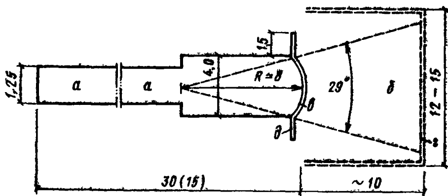
Рис. 8. План места для метания копья в «сетку» (размеры в метрах) \alpha — дорожка для бега; \beta — сектор для приземления снаряда; \gamma — планка; \delta — свободно выходящее ограждение. (В скобках приведено возможное уменьшение размеров)
