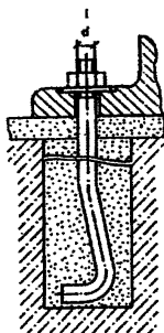
Рис.3. Болты, устанавливаемые в "колодях", заранее предусмот- ренных в фундаментах
