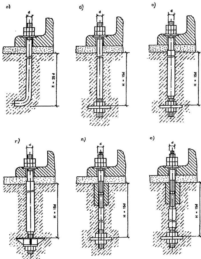
Рис.1. Болты, устанавливаемые в фундаменты до бетонирования а – изогнутые; б, в, г – с анкерной плитой; д, е – составные с анкерной плитой
