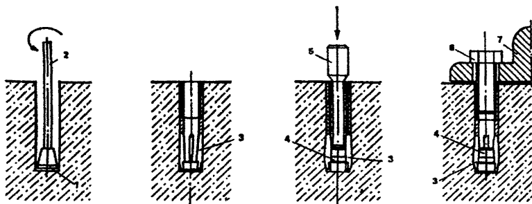
Рис.14. Технологическая схема установки долбель-штулки распорной 1 - коронка буровая; 2 - штанга буровая; 3 - распорная втулка; 4 - разжимная пробка; 5 - оправка; 6 - крепежный болт; 7 - обо- рудование
