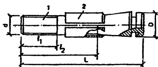
Рис.2 прил.1. Дюбель-шпилька распорная, тип 2
