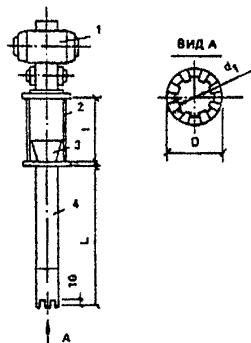
Рисунок прил.5. Уплотнительное устройство 1 - вибратор; 2 - удлинитель; 3 - воронка. 4 - уплотнитель; L - выполняется по максимальной высоте болта на объекте
