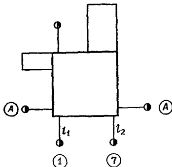
Рис. 14. Схема закрепления основных разбивочных осей здания размером 30×30 м
