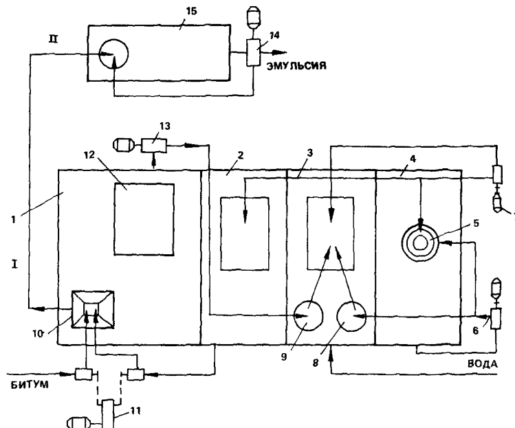
Рис. П1. Эмульсионная установка:
