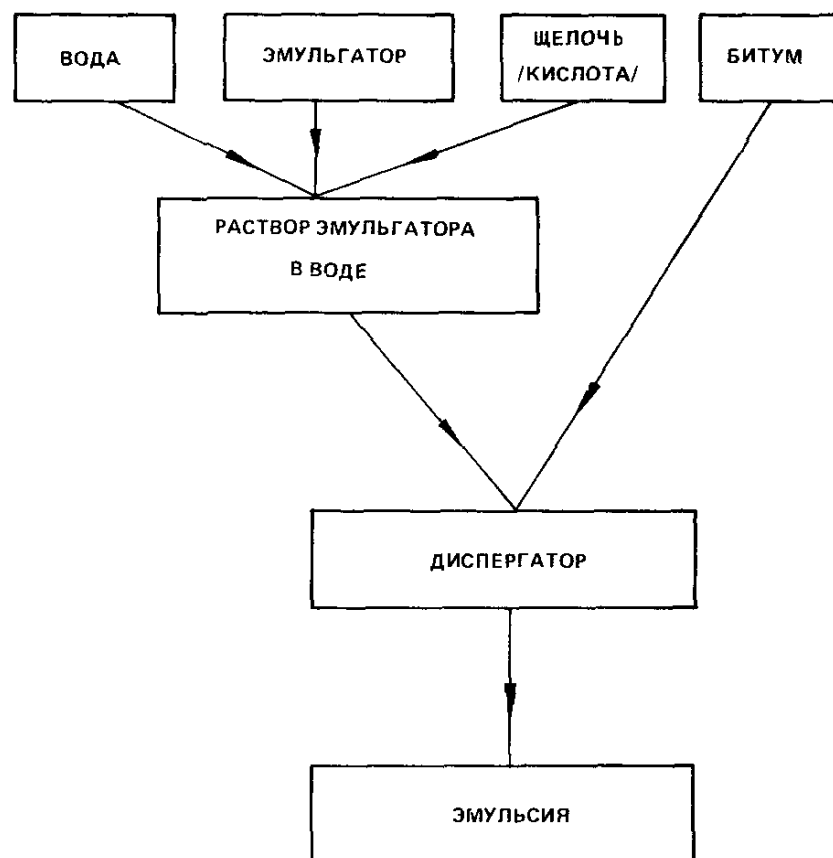
Рис. 1. Технологические схемы приготовления эмульсий
