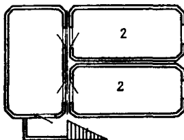
Рис. 1. Схема инвентарного дома-общежития из блок-контейнеров
