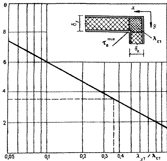
Рис.5. График для определения параметра \theta
