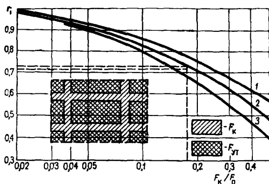
Рис.2. График для определения коэффициента \eta_1 при \lambda_{ут}/\lambda_k равном: 1 — 0,4; 2 — 0,3; 3 — 0,2
