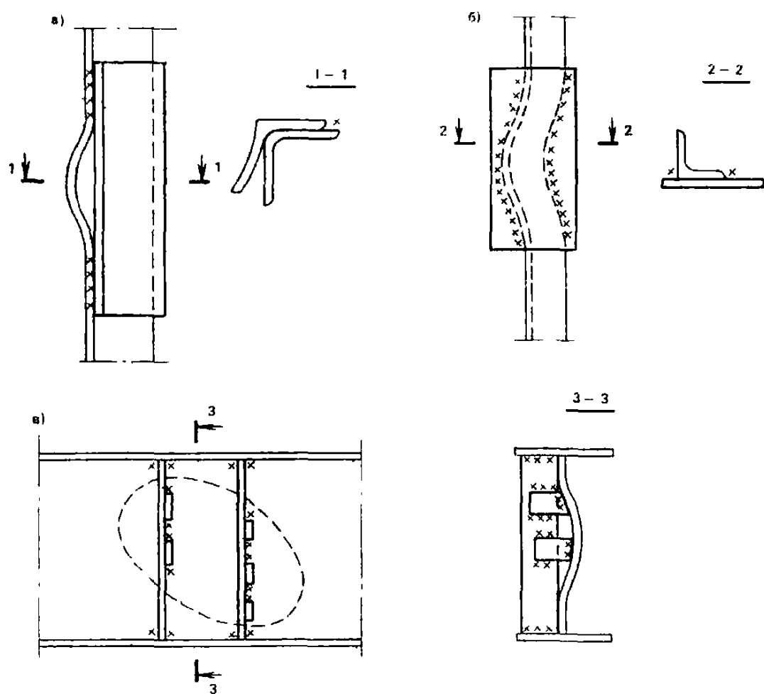
Рис. 33. Устранение дефектов в местах локальной погиби
