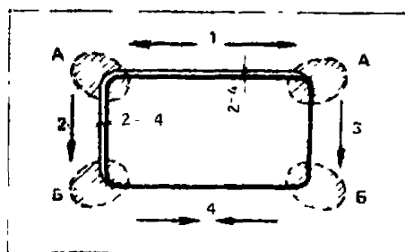
Рис. 32. Участки подогрева и последовательность сварки вставки
