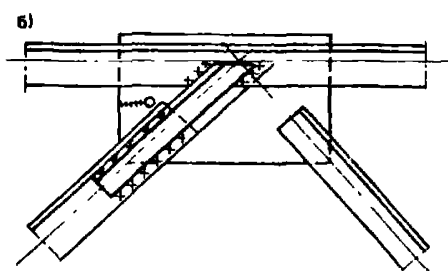
Рис. 27. Установка «энергетического мостика» для предотвращения распространения трещины а — до усиления, б — после заварки шва и усиления
