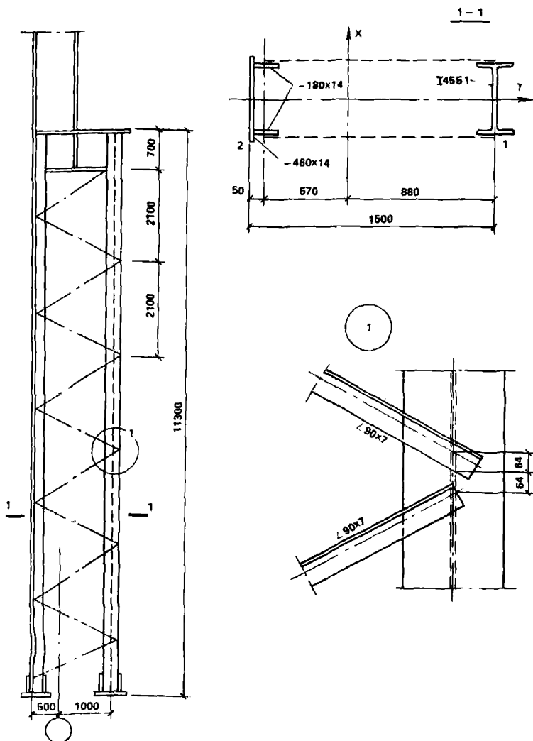
Рис. 3. К расчету (пример 5)
