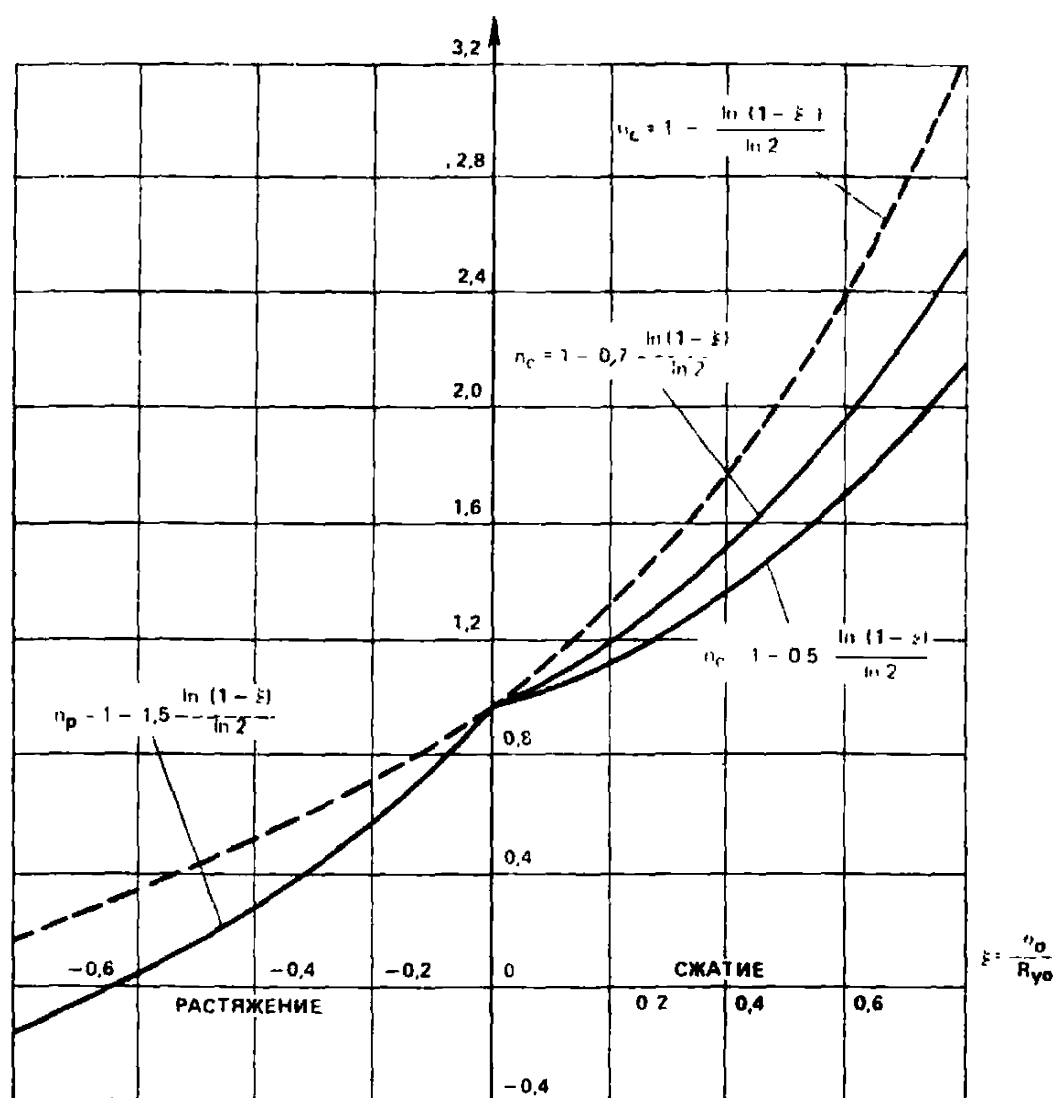
Рис. 17. Зависимости \eta(\xi) (сплошными линиями обозначены рекомендуемые значения, пунктирными — допусковые)
