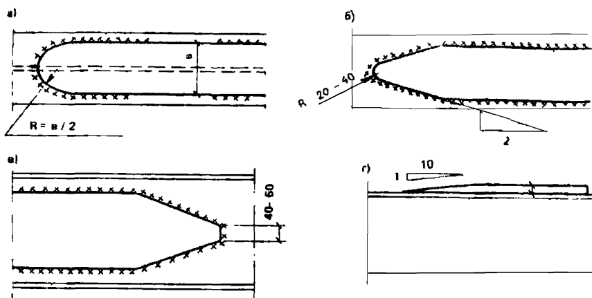
Рис. 26. Формы концов накладного листа
