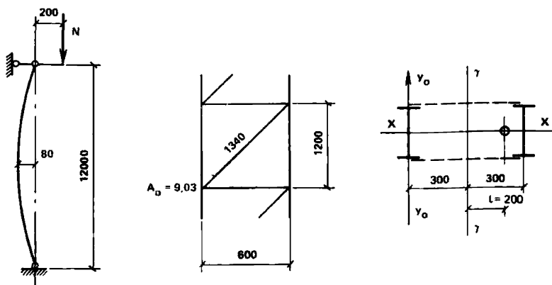
Рис. 2. К расчету (пример 4)
