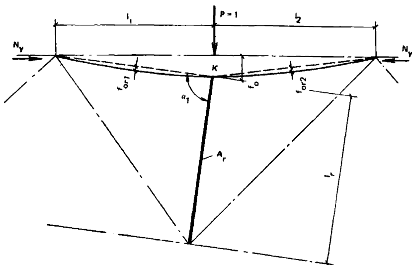
Ри. 22. Усиление сжатого элемента путем уменьшения расчетной длины
