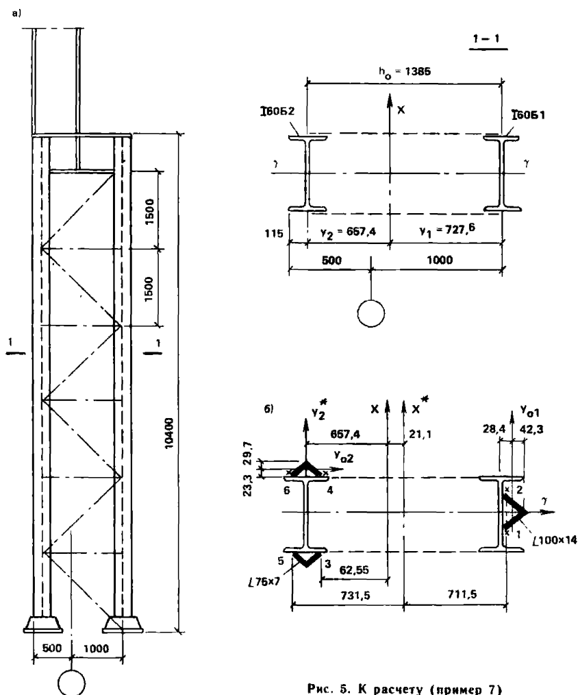
Рис. 5. К расчету (пример 7)
