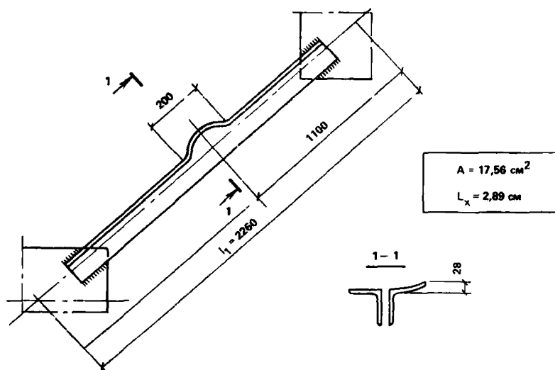
Рис. 1. К расчету (пример 3)
