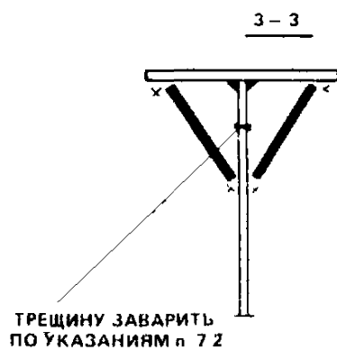
Рис. 30. Усиление верхней зоны подкрановых балок а--в -- варианты усиления
