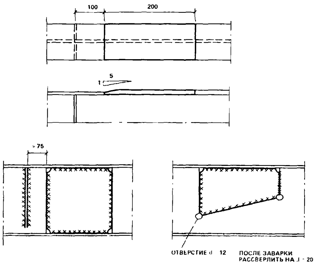
Рис. 25. Конструктивные требования к взаимному расположению швов
