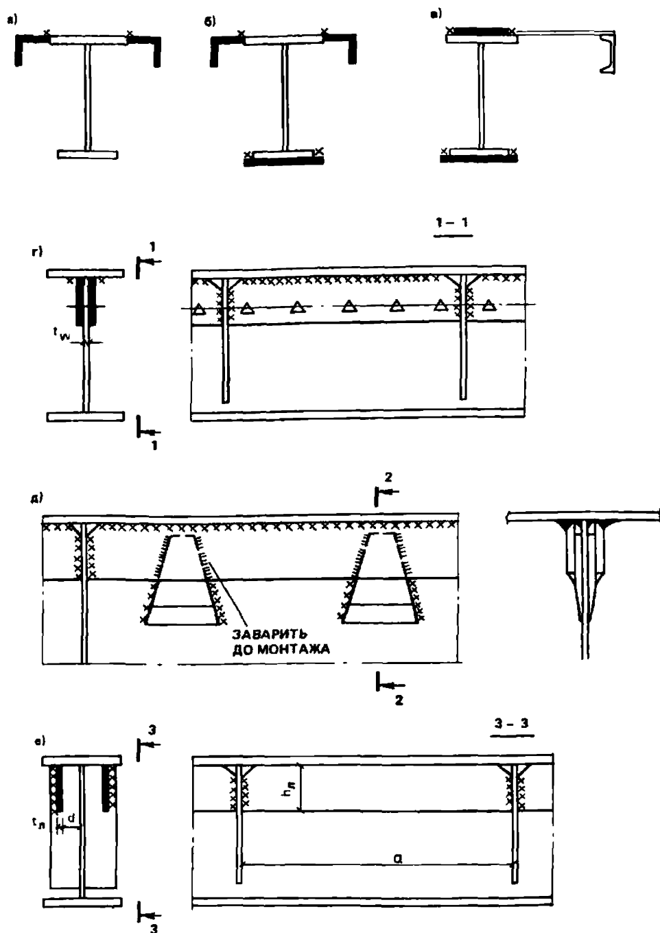
Рис. 6. Усиление подкрановых балок а—е — схемы усиления
