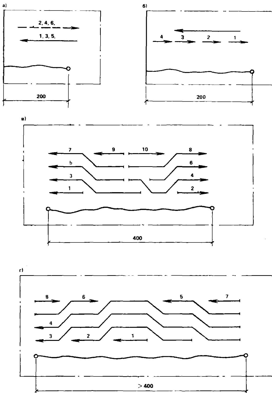
Рис. 29. Последовательность заварки трещины а, б — выходящих на свободную кромку; в, г — в средней части листа, 1—10 — последовательность наложения швов
