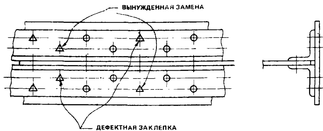
Рис. 34. Замена заклепок высокопрочными болтами
