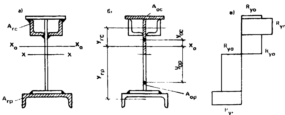
Рис. 18. К определению момента внутренних сил в усиленном сечении при развитии шарнира пластичности а — схема усиления, б — расположение сжатых (заштриховано) и растянутых зон в сечении, в — эпюр напряжений
