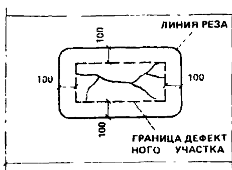
Рис. 31. Вырез дефектного участка
