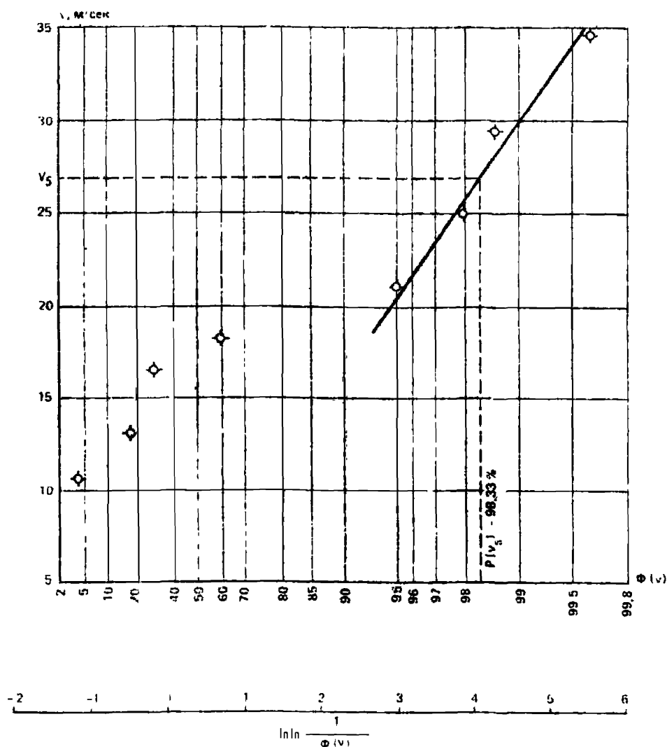
Рис. 2. Использование вероятностной бумаги распределения Гумбеля
