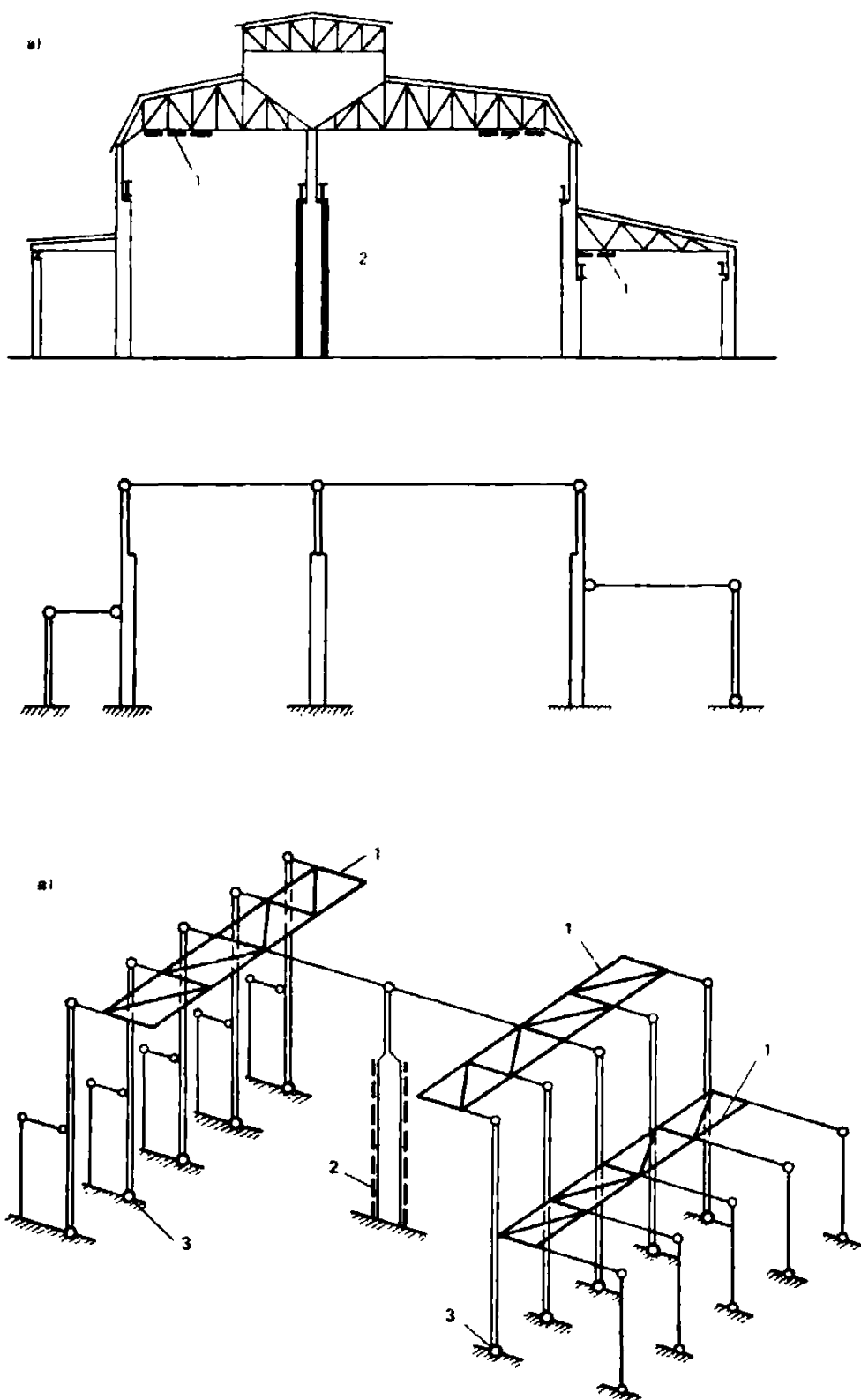
Рис. 13. Усиление путем введения в схему дополнительных элементов жесткости и шарниров а — поперечный разрез; б, в — расчетные схемы соответственно до и после усиления; 1 — элементы жесткости, 2 — увеличение сечений, 3 — шарниры
