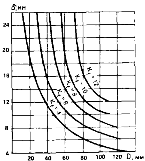
Рис. 24. Зависимость D от \sigma и k_f
