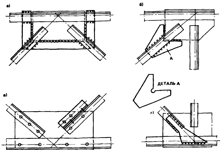
Рис. 8. Усиление узлов крепления стержней стропильных ферм
