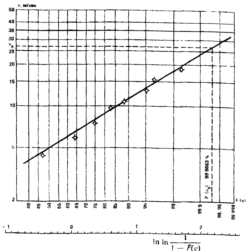
Рис. 1. Использование вероятностной бумаги распределения Вейбулла
