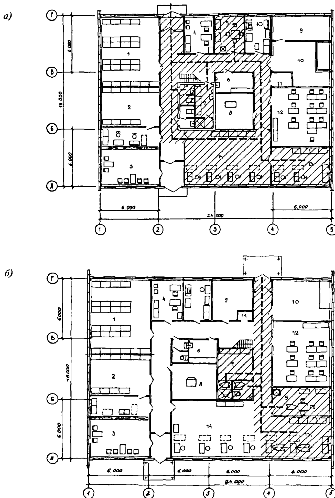
Черт. 6. Мастерская по ремонту бытовой радиоэлектронной аппаратуры
