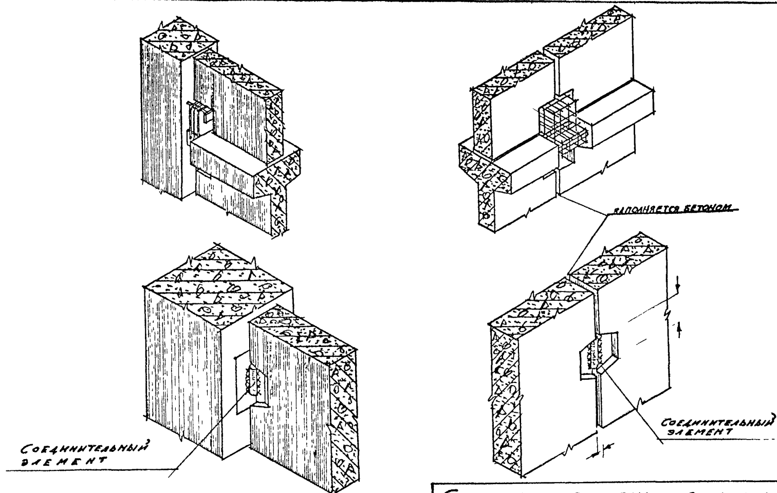
СХЕМА УЗЛОВ СОПРЯЖЕНИЯ ДИАФРАГМ ЖЕСТКОСТИ ПО СЕРИИ 1.020-2С
