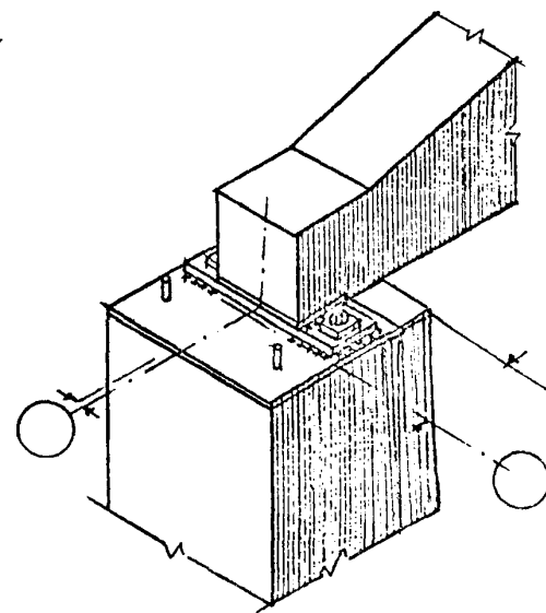
КРЕПЛЕНИЕ СТРОПНАБ- НОЙ ФЕРМЫ К КОЛОННЕ СРЕДНЕГО РЯДА
