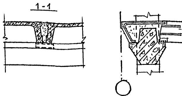
КРЕПЛЕНИЕ МЕЖКОЛОННЫХ ПЛАНТ ПОКРЫТИЯ К РИГЕЛЯМ У СРЕДНЕЙ КОЛОННЫ
