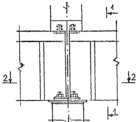
КРЕПЛЕНИЕ ПОДКРАНОВОЙ БАЛКИ НА КОНСОЛ КАРНИЗЫ
