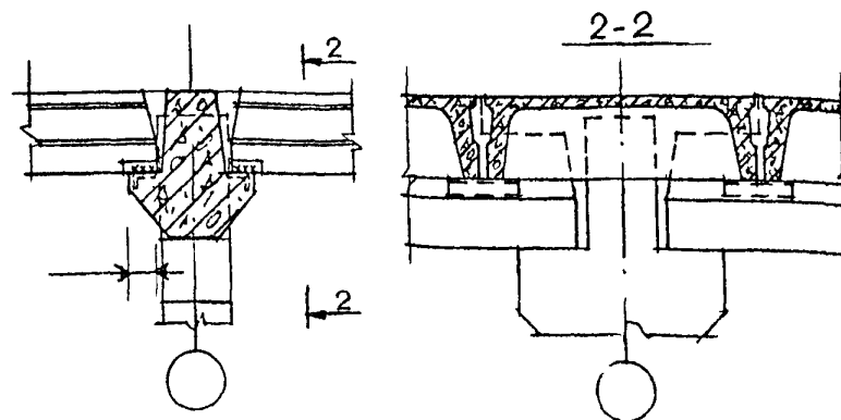
СХЕМА УЗЛОВ КРЕПЛЕНИЯ ПЛАНТ ПЕРЕКРЫ- ТИЯ И СОПРЯЖЕНИЯ МЕЖКОЛОННЫХ ПЛАНТ ПЕРЕКРЫТИЯ И ПОКРЫТИЯ
