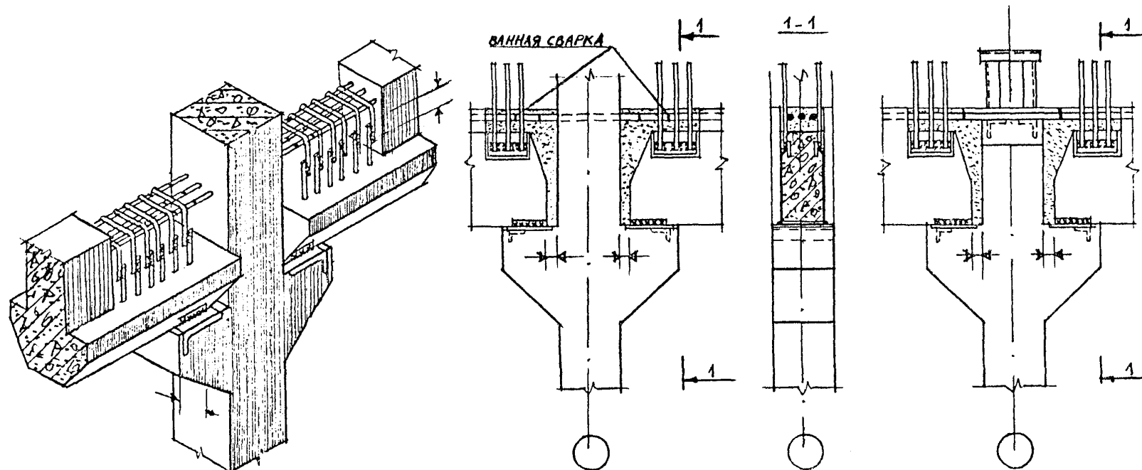
СОПРЯЖЕНИЕ РИГЕЛЕЙ ПОКРЫТИЯ СО СРЕДНЕЙ КОЛОННОЙ
