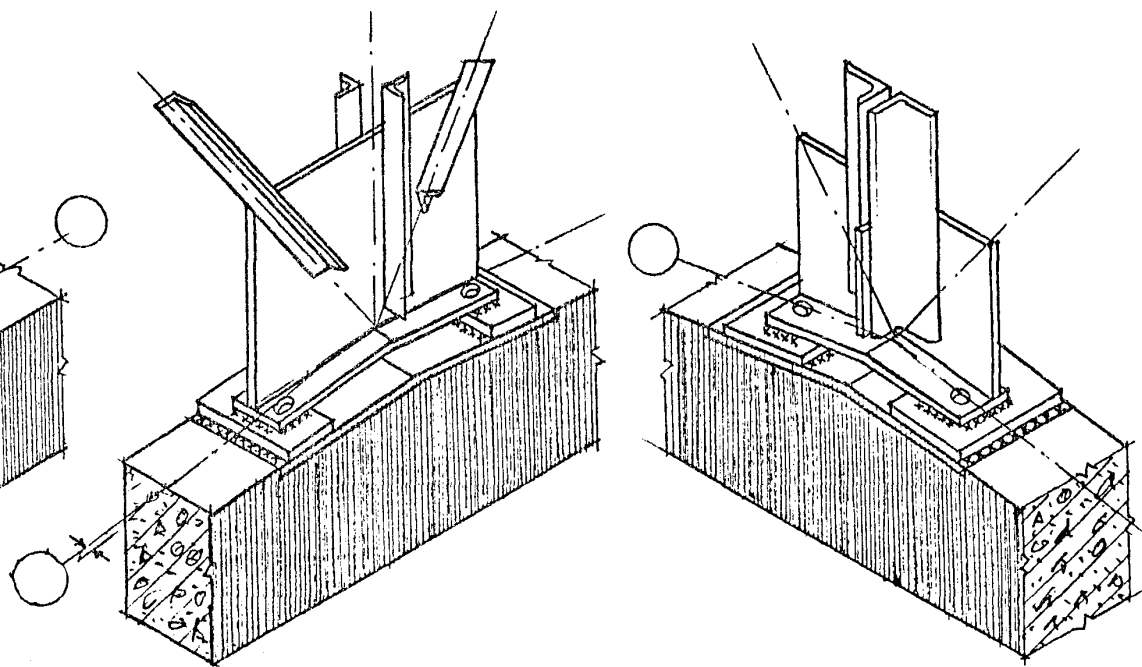
КРЕПЛЕНИЕ СРЕДНИХ СТОЕК ФЕРМ ФОНАРЯ
