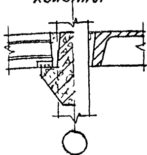
КРЕПЛЕНИЕ МЕЖКОЛОН- НЫХ ПЛАНТ ПЕРЕКРЫТИЯ К РИГЕЛЯМ У СРЕДНЕЙ КОЛОННЫ
