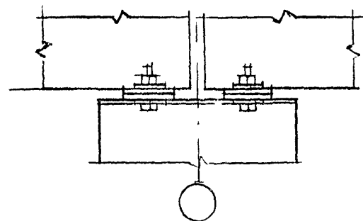
СХЕМА УЗЛОВ СОПРЯЖЕНИЯ ПОДКРАНОВЫХ БАЛОК И СТРОПЬЯВНЫХ КОНСТРУКЦИЙ С КОЛОННАМИ В СЕЙСМИЧЕСКИХ РАЙОНАХ
