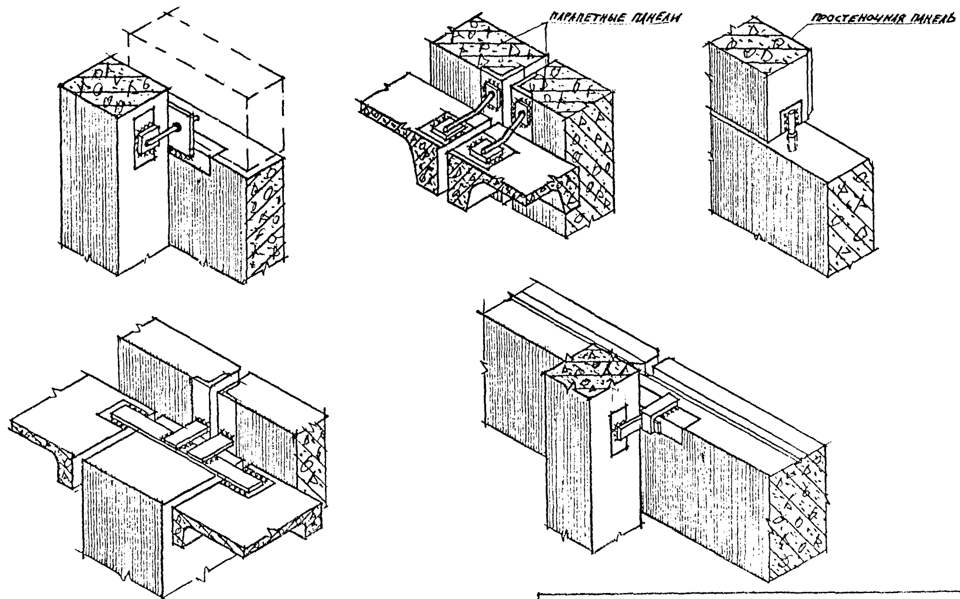
СХЕМА УЗЛОВ ХРЕПЛЕНИЯ ПАНЕЛЕЙ СТЕНОВОГО ОГРАЖДЕНИЯ
