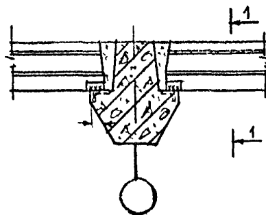
КРЕПЛЕНИЕ РЯДОВЫХ ПЛАНТ ПОКРЫТИЯ И ПЕРЕКРЫТИЯ К РИГЕЛЯМ РЯДОВЫХ РАМ
