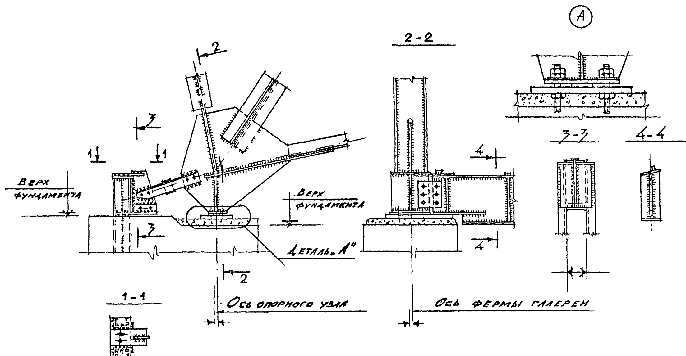
СХЕМА УЗЛА ФЕРМЫ ТРАНСПОР- ТЕРНОЙ ГАЛЕРЕИ
