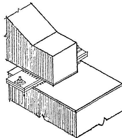
СОПРЯЖЕНИЕ СТРОПЬЯВ- НОЙ КОНСТРУКЦИИ С КОЛОННОЙ
