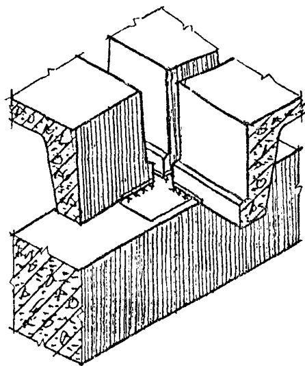
ОПИРАНИЕ ПЛИТ НА РЯДОВУЮ ФЕРМУ
