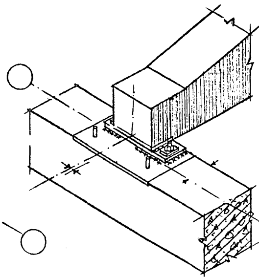
ОПИРАНИЕ СТРОПНАБНОЙ ФЕРМЫ В СЕРЕДИНЕ ПРО- ЛЕТА ПОДСТРОПНАБНОЙ ФЕРМЫ
