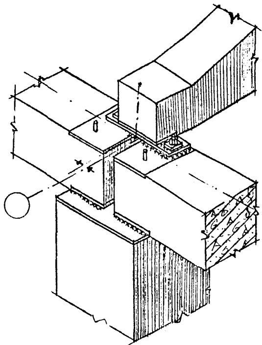
ОПИРАНИЕ ПОДСТРОПНАБНЫХ ФЕРМ НА КОЛОННУ И СТРОПНАБ- НОЙ ФЕРМЫ НА ПОДСТРОПНАБНЫЕ
