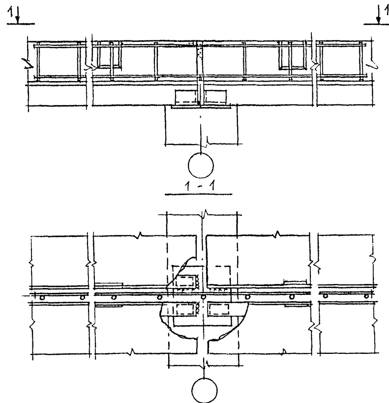
СХЕМА СОПРЯЖЕНИЯ ПИЛТ ПОКРЫТІЯ СО СТРОПНАВНИМИ КОНСТРУКЦІЯМИ
