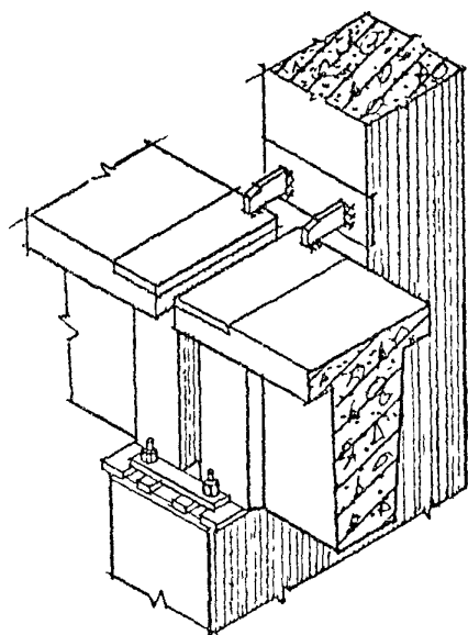
КРЕПЛЕНИЕ ПОДКРАНОВОЙ БАЛКИ НА КОНСОЛ КАРНИЗЫ
