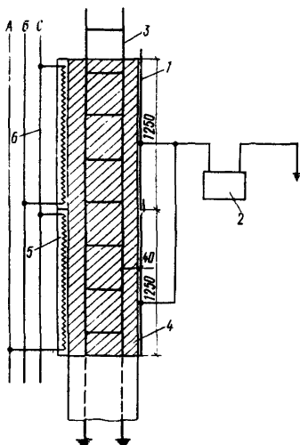
Рис.6. Схема комбинированного электровоздействия при термообработке бетона по методу КЭВ
