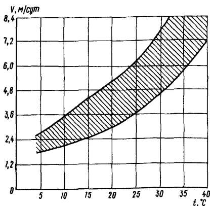
Рис.1. График зависимости скорости подъема скользящей опалубки V от температуры t^\circ наружного воздуха
