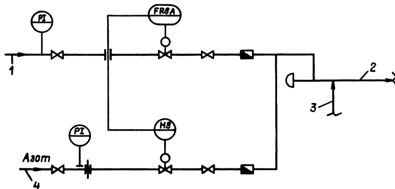
Принципиальная схема подачи продувочного газа в факельный коллектор
