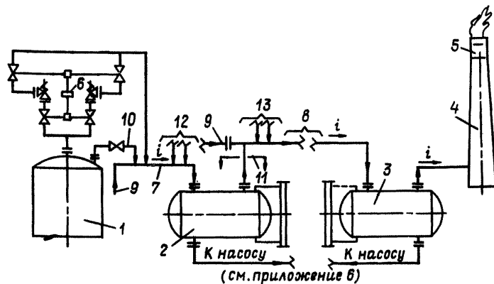
Принципиальная схема сброса газов (паров) в факельную систему от предохранительных клапанов
