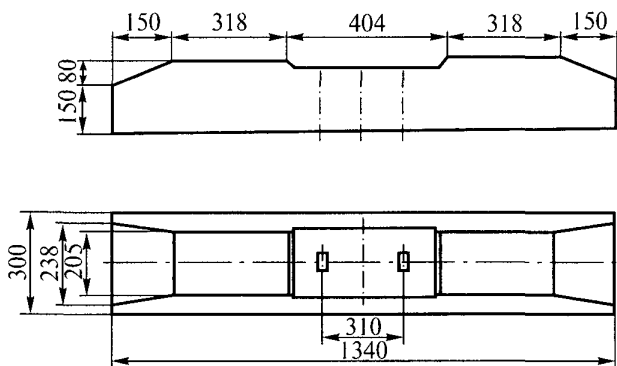
Рис. П.10.2. Железобетонная полупала ПШН1-13-325-1
