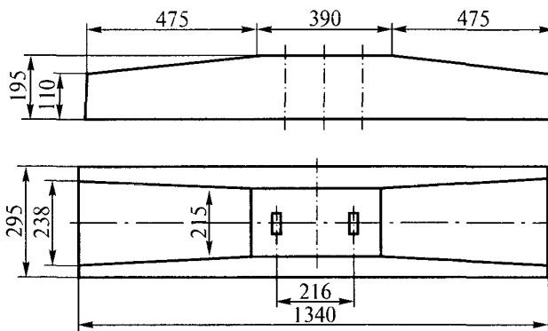
Рис. П.10.3. Железобетонная полупала ПШН4-13-325-1
