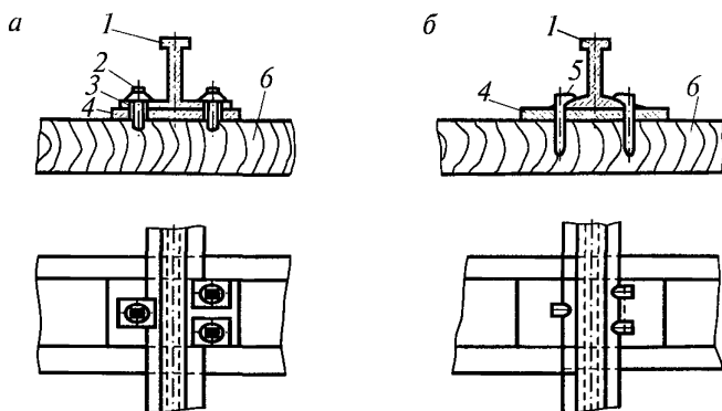
Рис. П.10.5. Прикрепление рельсов к полушпалам: а — шурупами; б — костылями; 1 — рельс; 2 — шуруп путевой; 3 — прижим; 4 — подкладка; 5 — костыль путевой; 6 — полушпала
