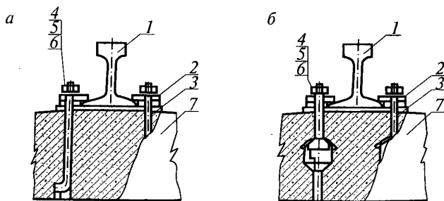
Рис. П.10.6. Прикрепление рельсов к железобетонным элементам разъемное: а — с нестандартным закладным болтом; б — со стандартным закладным болтом по ГОСТ 16017; 1 — рельс; 2 — прижим; 3 — упругая прокладка; 4 — болт; 5 — гайка; 6 — шайба; 7 — железобетонный подрельсовый опорный орган
