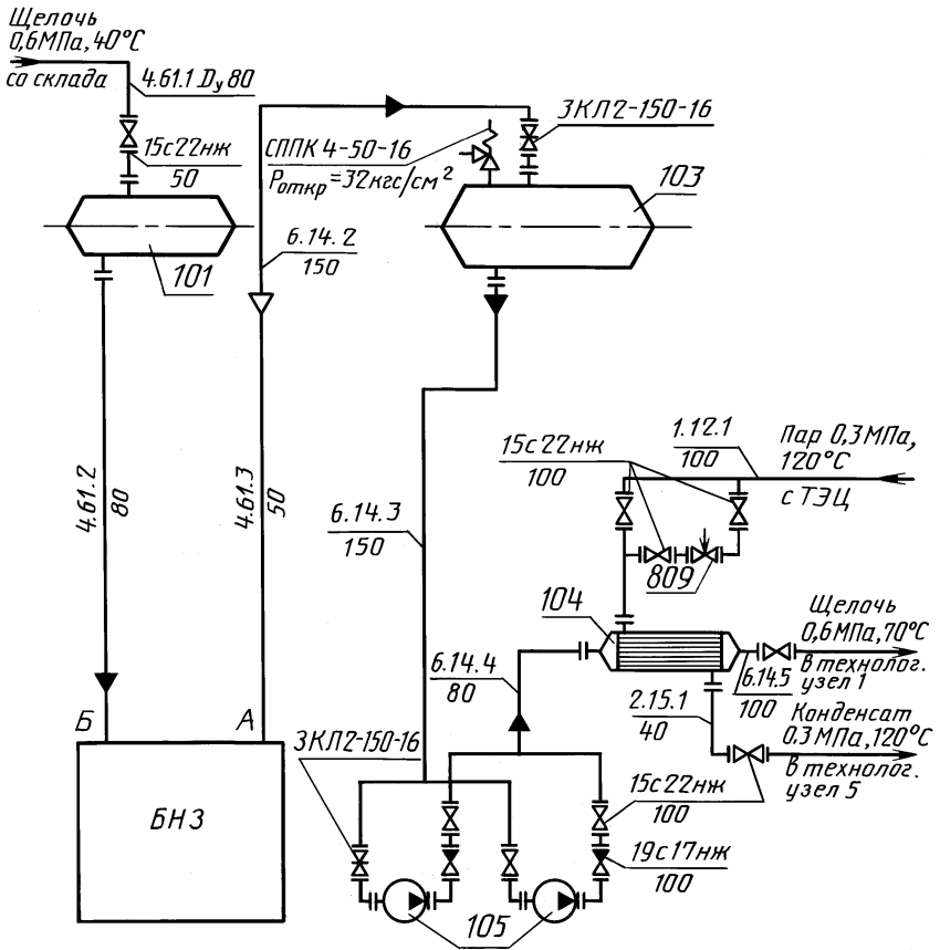
Схема соединений (монтажная)
