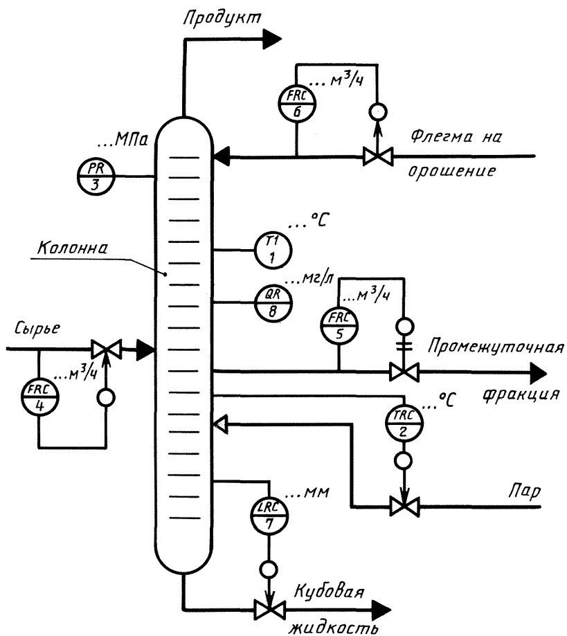
Пример выполнения схемы автоматизации упрощенным способом
