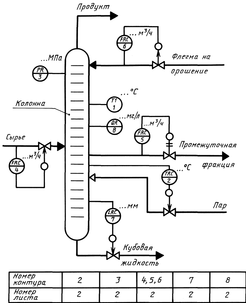
Пример выполнения схемы автоматизации упрощенным способом
