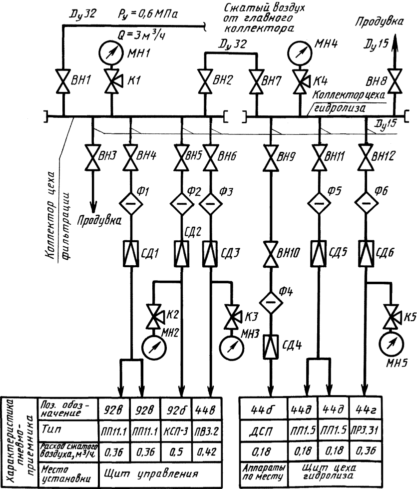
Пример выполнения принципиальной схемы пневмопитания
