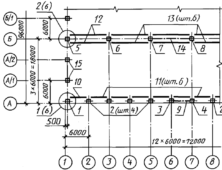
Схема расположения колонн и подкрановых балок
