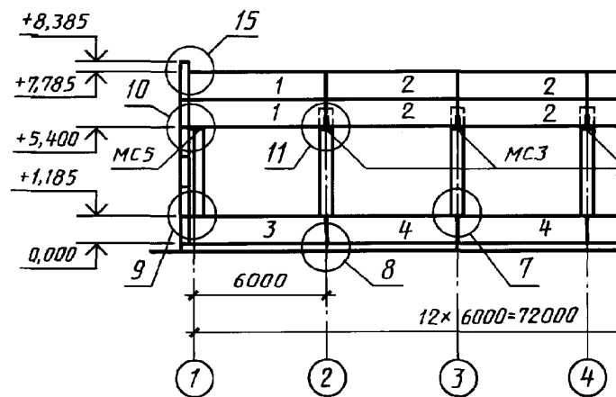
Схема расположения панелей стен
