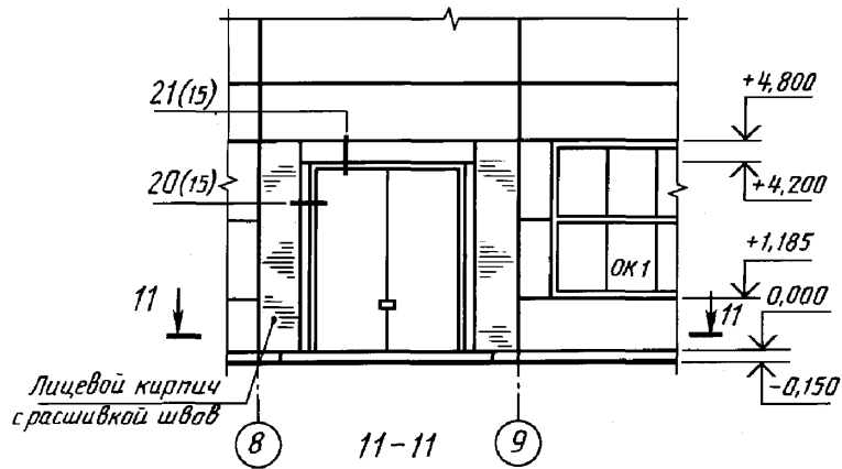
Фрагмент 3 фасада
