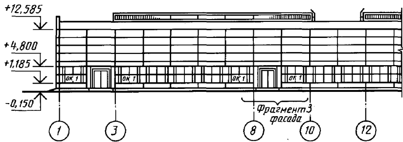
Фрагмент 3 фасада
