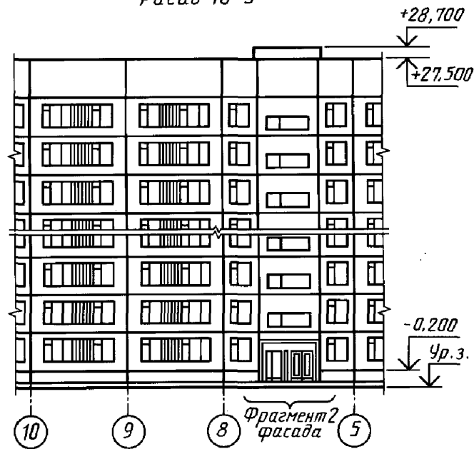
Фасад 10-5
