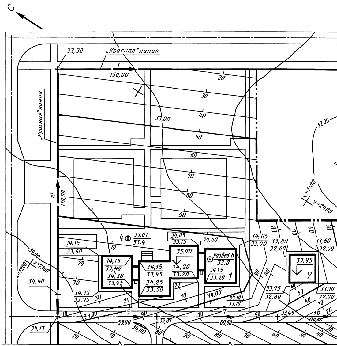
Пример оформления плана организации рельефа в проектных горизонталях
