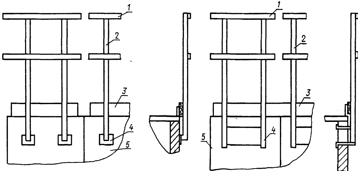
1 — заполнение; 2 — стойка; 3 — бортовая доска; 4 — место крепления (к стене или за оконный проем); 5 — стена здания
