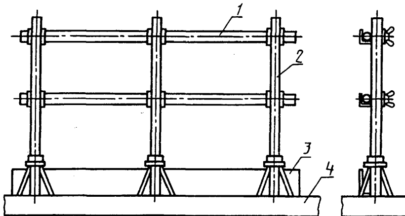
1 — заполнение; 2 — стойка; 3 — бортовая доска; 4 — плита перекрытия
