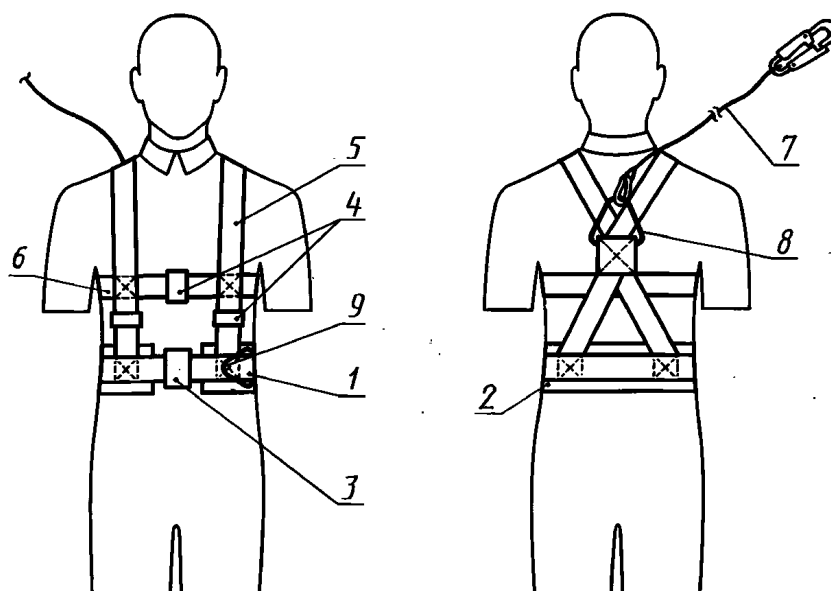
Рисунок 3 — Лямочный пояс , тип В
