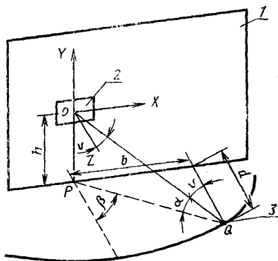
1 — наружная стена; 2 — испытываемый образец; 3 — громкоговоритель
