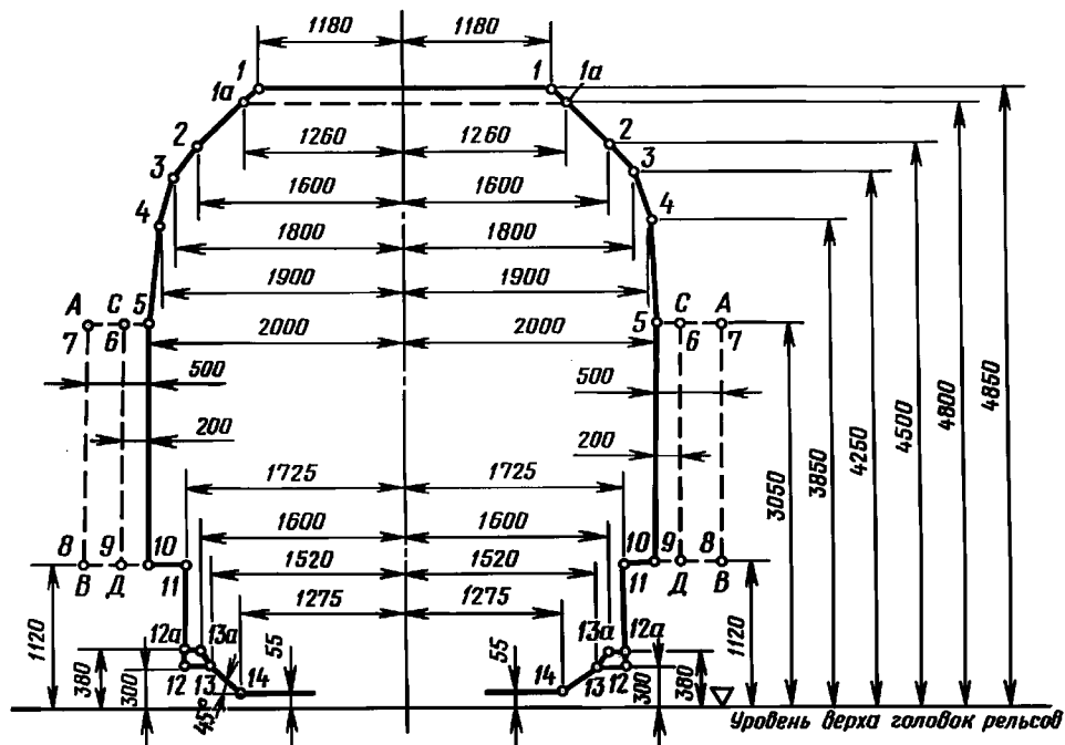
Габарит 1-СМ Верхнее очертание габарита
