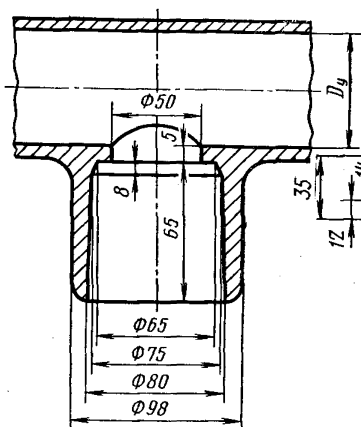
Раструб типа III
