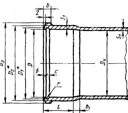
Раструб типа II
