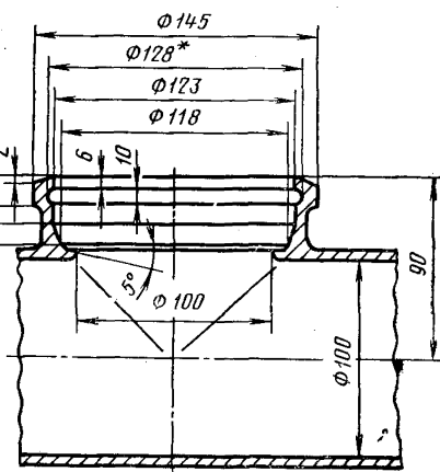
Раструб типа IV
