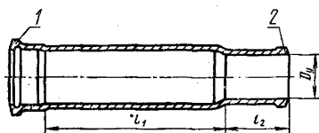
1 — раструб типа II по ГОСТ 6942.2—80; 2 — хвостовик по ГОСТ 6942.2—80
