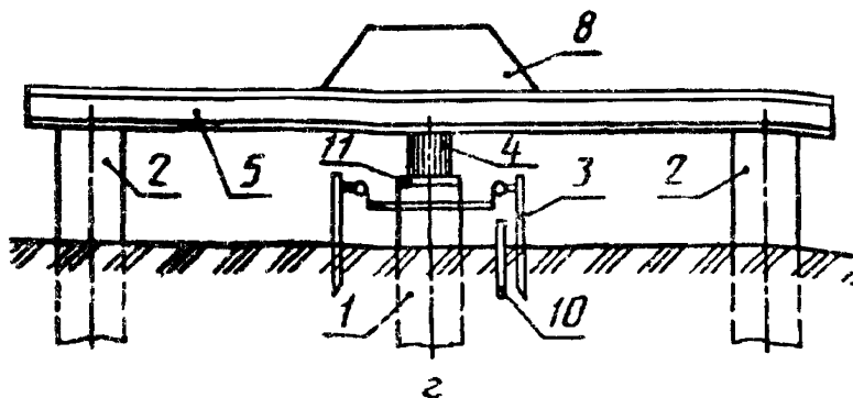
Установка комбинированная
