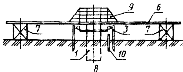
Установка комбинированная
