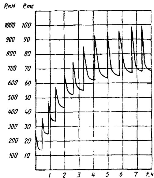
Рисунок 2 — График релаксации нагрузки за время испытания
