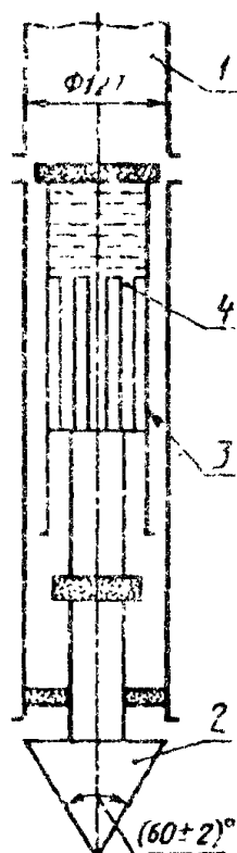
1 — труба (ствол сваи), 2 — наконечник; 3 — муфта трения, 4 — гидроцилиндр
