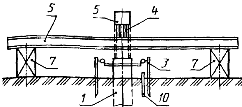
Схема установки для испытания грунтов статической выдергивающей нагрузкой
