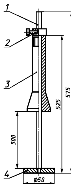
1 — направляющая; 2 — фиксатор; 3 — падающий груз; 4 — наковалья
