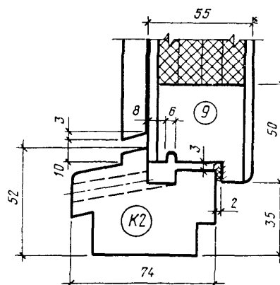
б) По нижнему притвору
