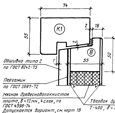
а) По верхнему притвору
