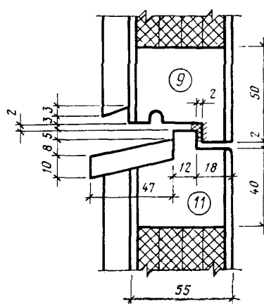
г) По среднему притвору
