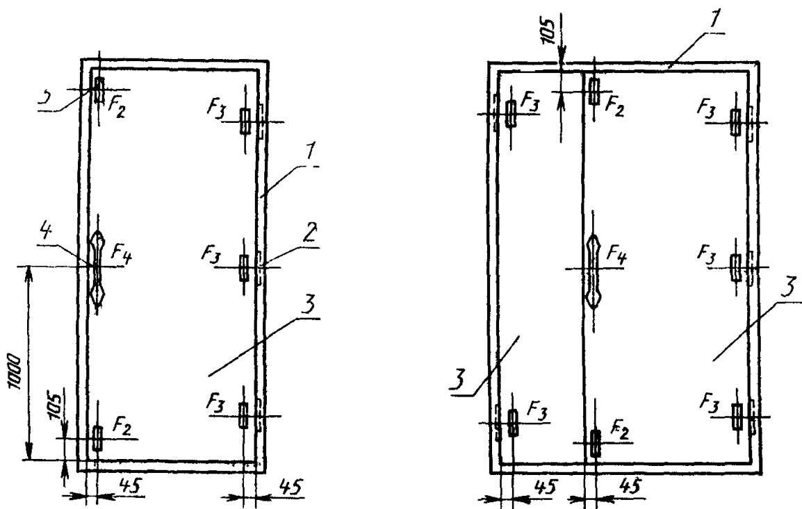
Рисунок 2 — Схема испытаний статическими нагрузками F_2 , F_3 , F_4
