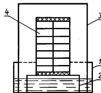
Ванна с гидравлическим затвором
