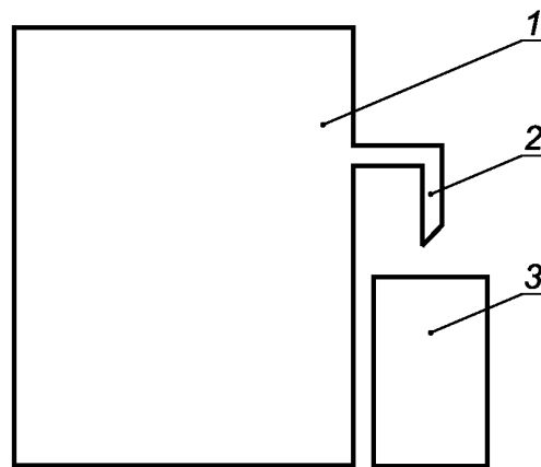
1 — сосуд; 2 — трубка; 3 — емкость для сбора воды
