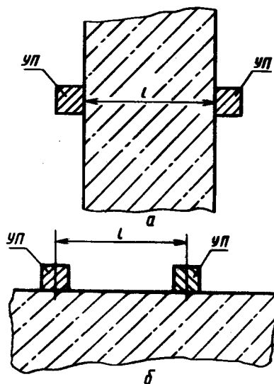
a — схема испытания бетона способом сквозного прозвучивания; б — схема испытания бетона способом поверхностного прозвучивания; УП — ультразвуковые преобразователи; l — база прозвучивания
