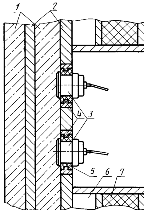
1 — бетон; 2 — разделительные листы кассеты; 3 — преобразователи; 4 — рабочие поверхности преобразователей; 5 — акустическая изоляция; 6 — паровая рубашка; 7 — теплоизоляция
