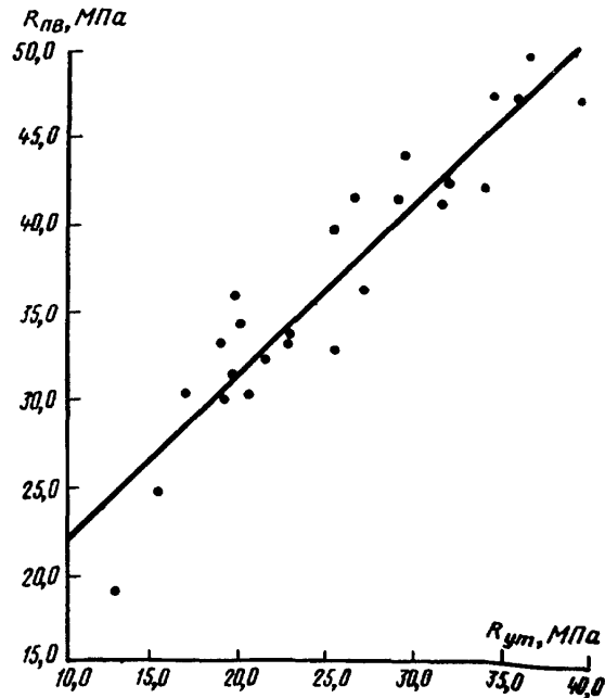
График градуировочной зависимости
