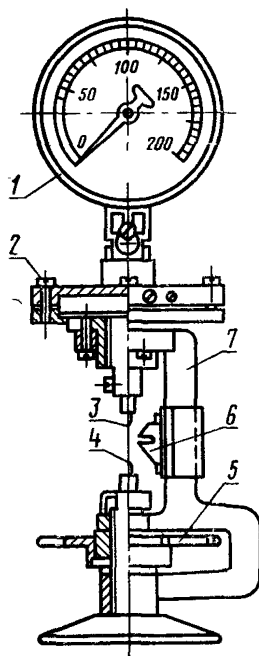
1 — манометр; 2 — гидравлическая пресса; 3 — верхний зуб; 4 — нижний зуб; 5 — щелевой упор; 6 — диск винтового механизма; 7 — корпус прибора
