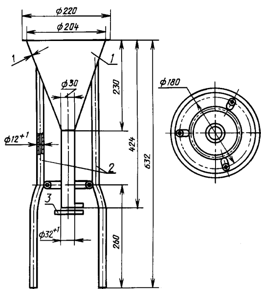
Воронка для определения насыпной плотности песка
