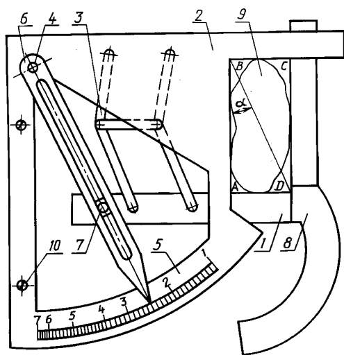
Формометр
