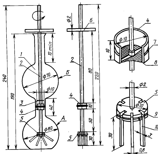
Плотномер ДКП-2
