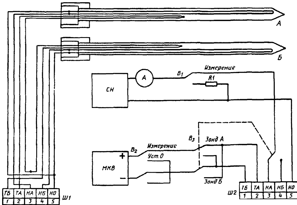
Рисунок 1 — Устройство зонда и электрическая схема соединения приборов
