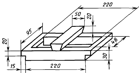
Опорная планка
