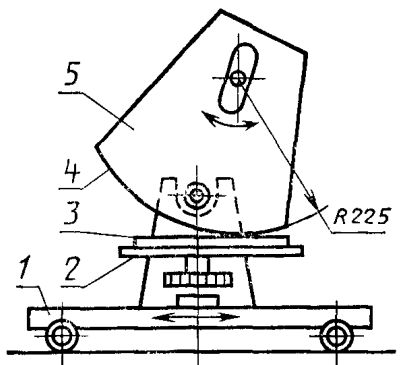
1—площадка; 2—стол, 3—образец; 4—шлифовальная шкурка, 5—рабочий элемент
