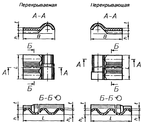
Рисунок 2 — Коньковые детали
