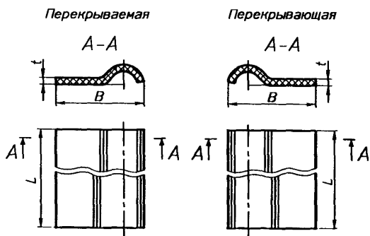
Рисунок 3 — Упрощенные коньковые детали
