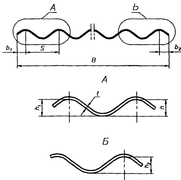
Рисунок 1 — Форма поперечного сечения волнистого листа
