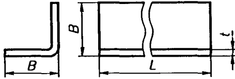
Рисунок 4 — Равнобокая угловая деталь
