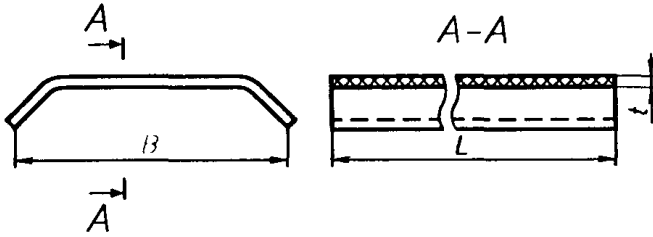
Рисунок 5 — Лотковая деталь
