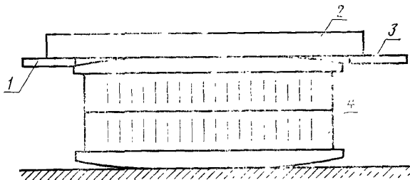
1 — щуп первый; 2 — поверочная линейка; 3 — щуп второй; 4 — блок
