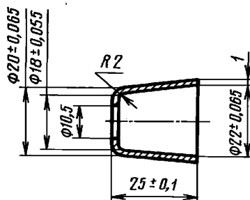
Колшачок для кельм и лопаток
