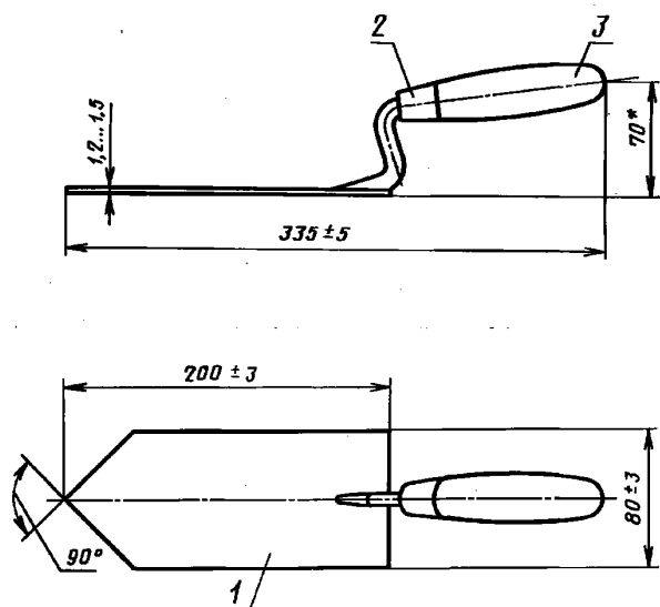
Лопатка типа ЛК
