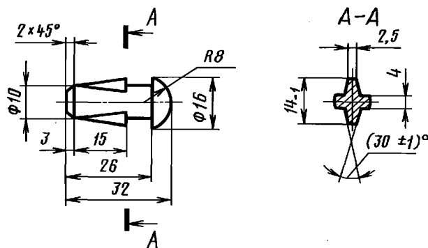
Грибок для кельм типов КБ и КП
