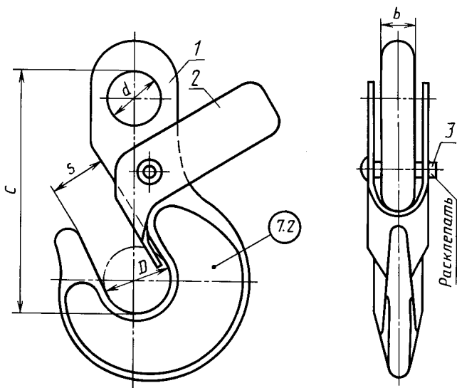
1 — крюк; 2 — замок; 3 — заклепка
